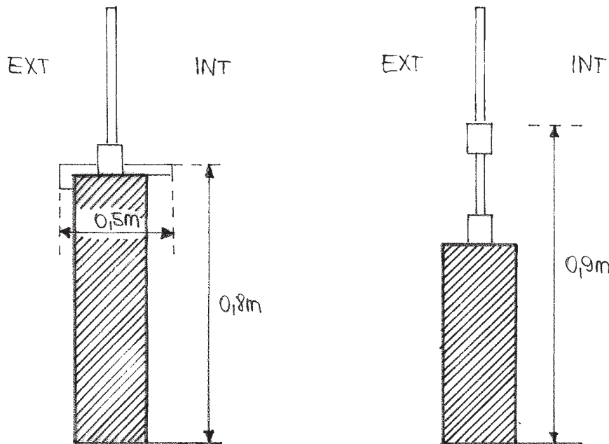
Figure 17 Hauteurs allèges
