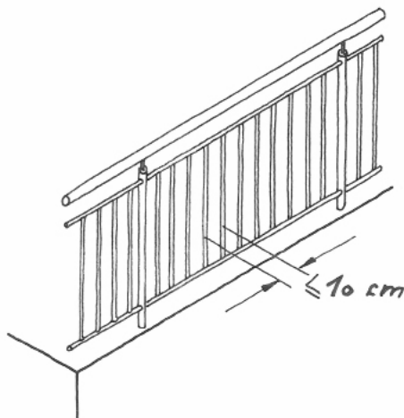
Figure 16 Géométrie des garde-corps (entraxe entre barreaux verticaux et dispositif empêchant d'y grimper)
