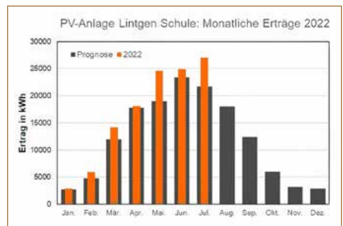
Ab. 2: Monatliche Erträge der Photovoltaikanlage auf dem Dach der Grundschule in Lintgen
